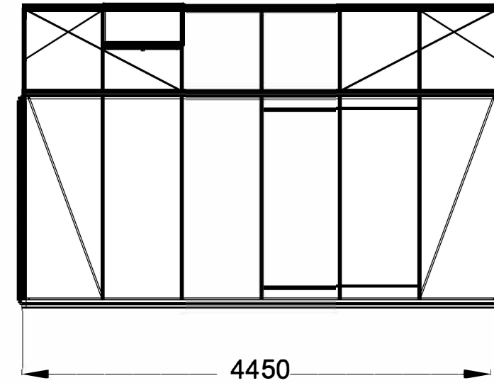
Right/leftview
