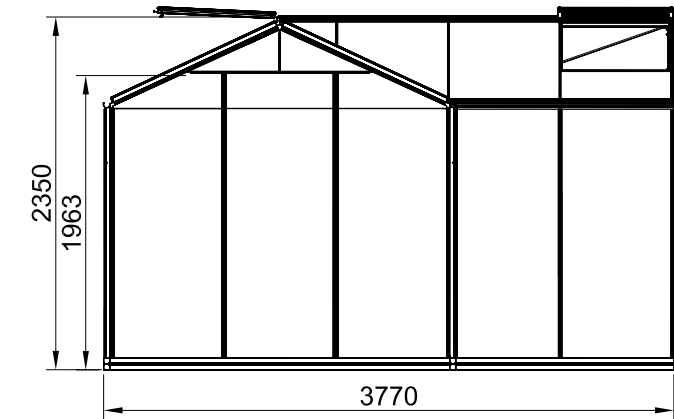
Right/leftview
